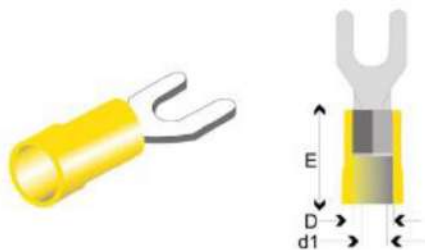
Terminal Aislada Horqueta Amarilla
