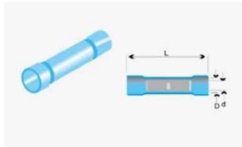
Terminal Termoencogible Vinilo Tubular
