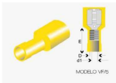
Terminal Aislado Fanton Hembra M5 - 6.4V
