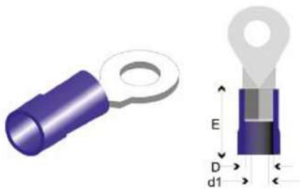
Terminal Aislado Aro Azul
