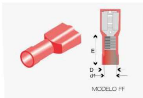
Terminal Aislado Faston Nylon Hembra
