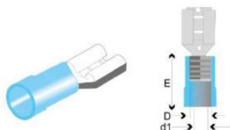
Terminal Faston Termoencogible Hembra
