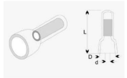
Terminal Aislado Conector de Ponchar
