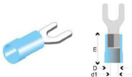
Terminal Termoencogible Horqueta Azul
