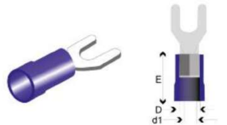
Terminal Aislada Horqueta Azul
