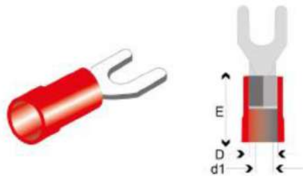
Terminal Aislada Horqueta Roja
