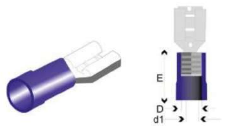
Terminal Aislada Faston Hembra Azul
