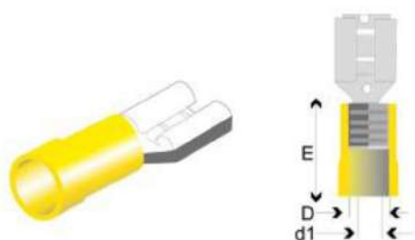
Terminal Aislado Faston Hembra Amarillo
