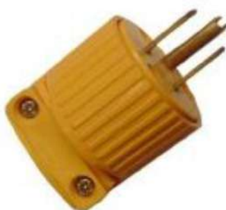
Clavija 3P x 15Amp Amarillo
