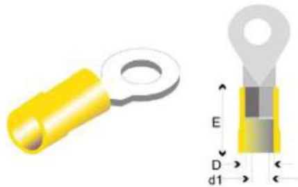
Terminal Aislado Aro Amarillo
