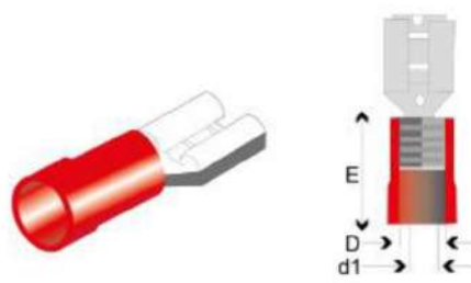
Terminal Aislada Faston Hembra rojo
